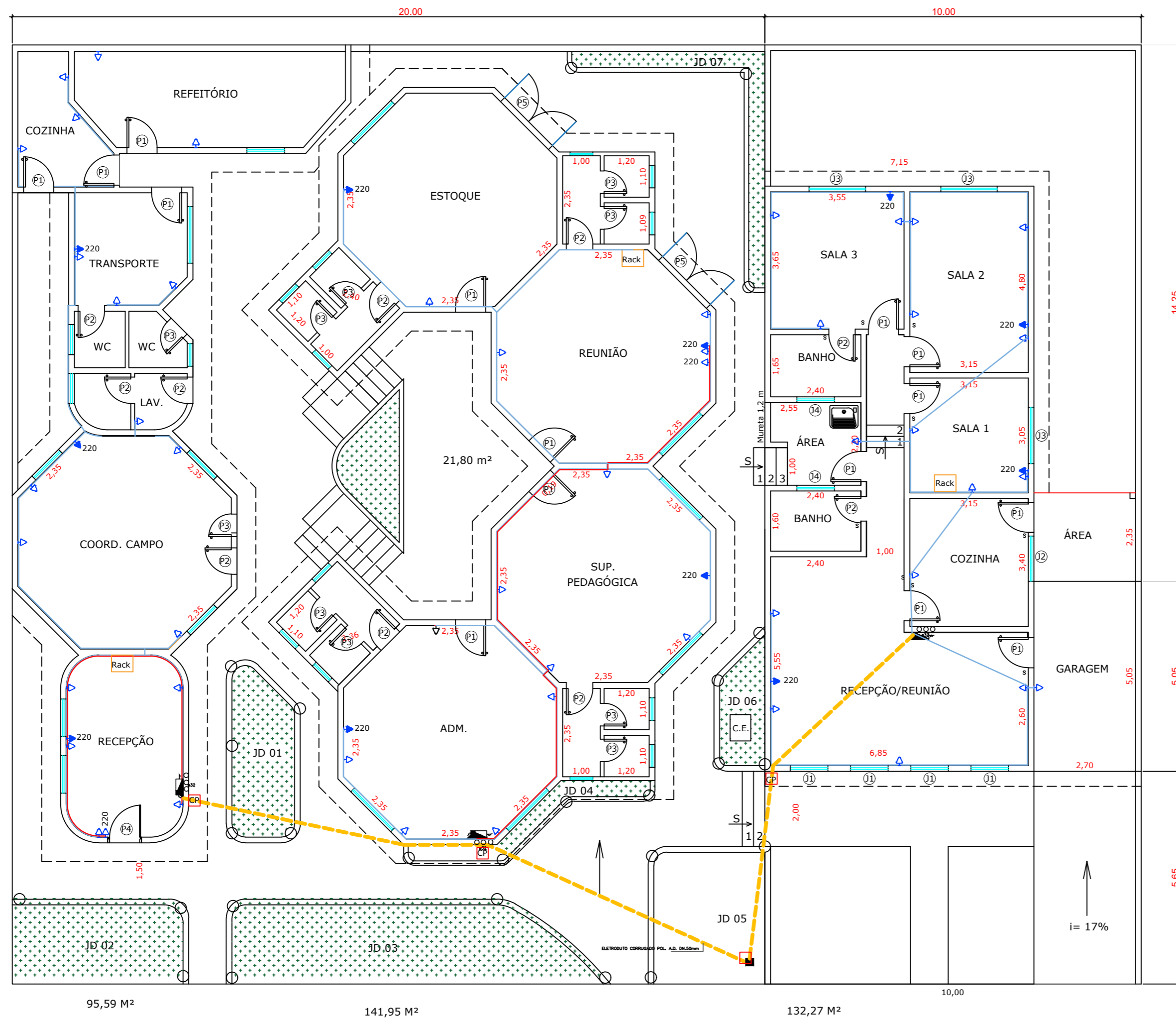
PLANTA BAIXA- ELÉTRICA ESC. 1:100
